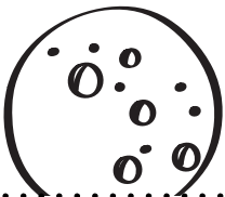
Moon
