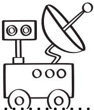
Mars rover
